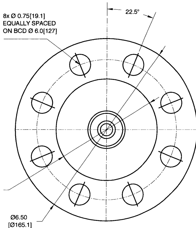
2" ANSI 600 # RF FLANGE
